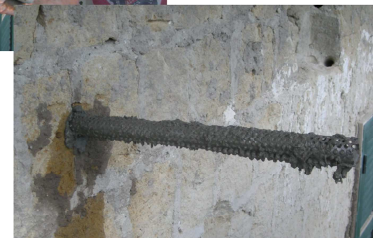
inserimento del paletto "PERFO" nel foro
