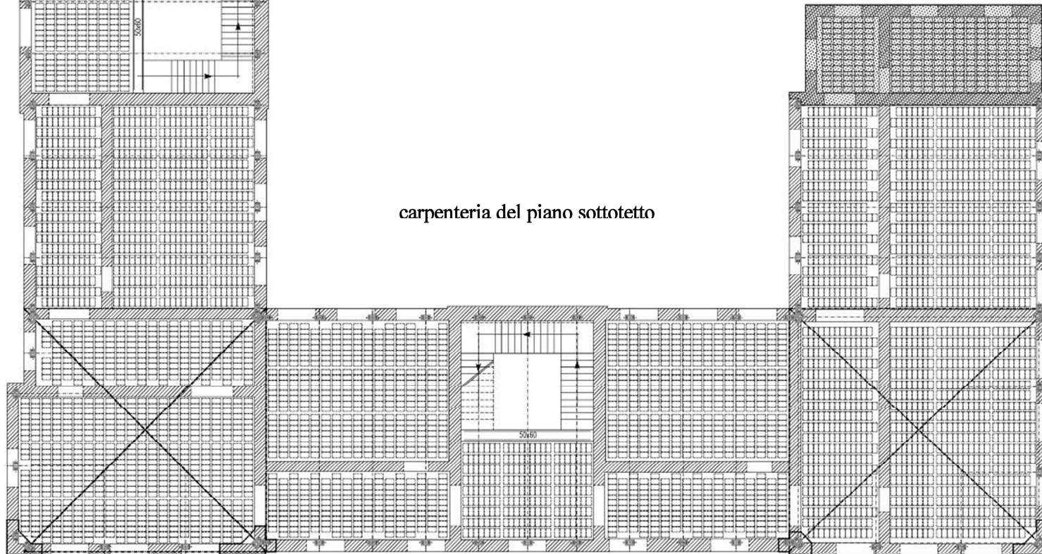
soffitto armato
