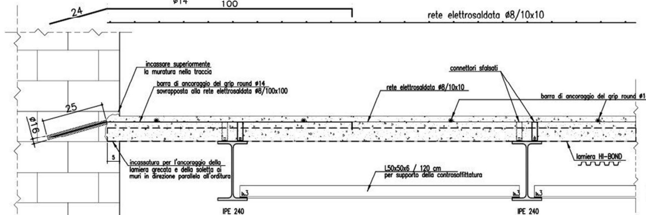
sezione trasversale al verso di orditura
