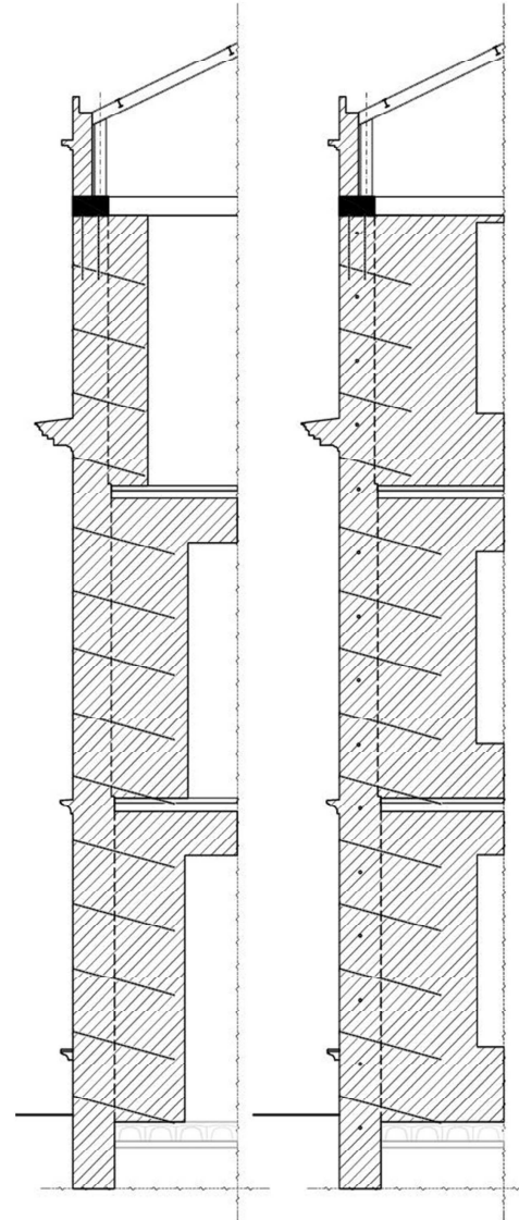
sezione chiodature orizzontali
