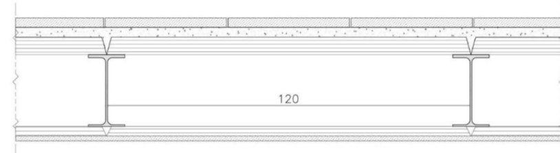
Sezione trasversale del solaio preesistente
