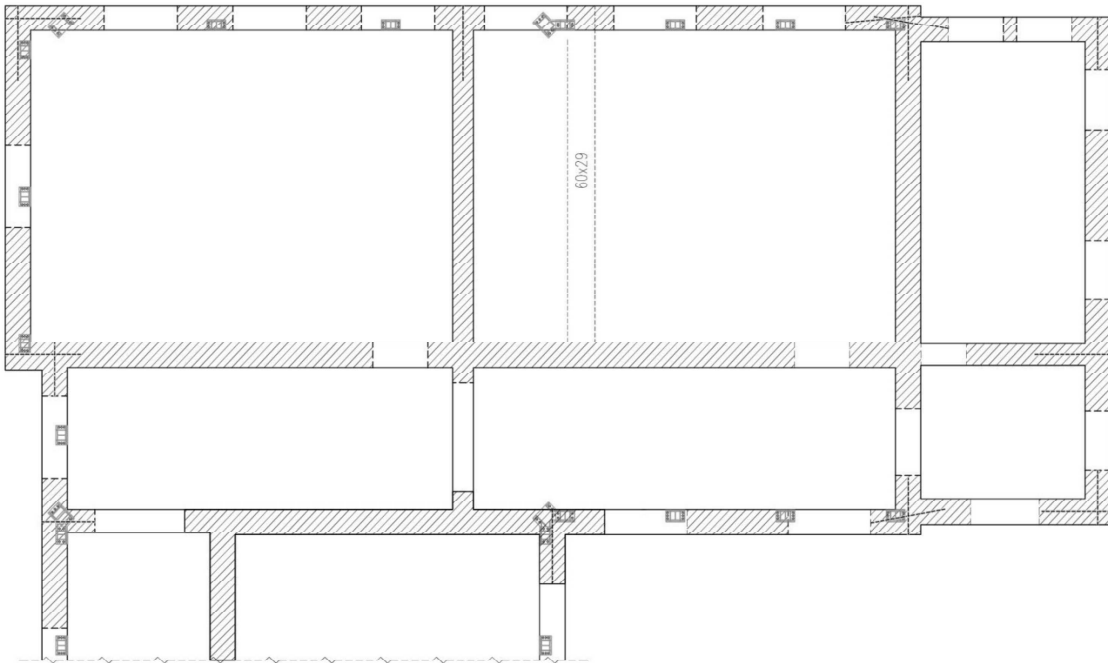
stralcio di carpenteria delle chiodature orizzontali
