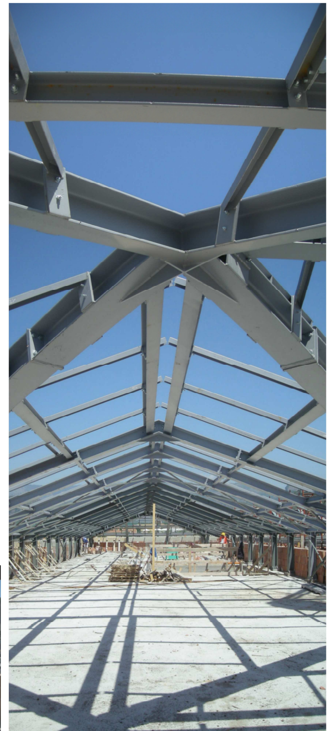
lo sviluppo longitudinale della copertura
